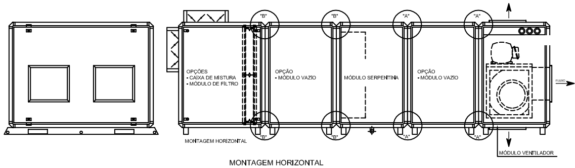
Fig. XVII - 16 - Montagem Horizontal 05 a 50 - DX/DL
