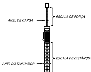
Fig. XV-01 - Medidor de tensão da correia
