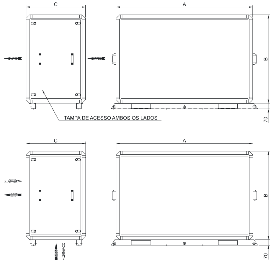
Fig. XVII 01 - Cotas Módulo Vazio 05 a 50 (DX e DL)
