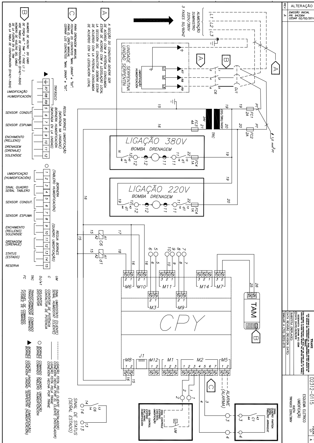
Fig.XVIII-03 - Esquema elétrico de Força e Comando (Umidificação) - 220/380V (trifásico)
