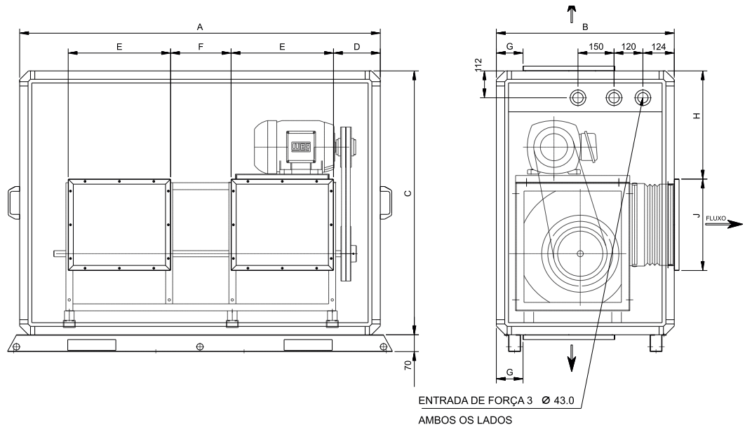
Fig. XVII-07 - Dimensões Módulo Ventilador 12,5 a 30 - Siroco e Limit Load
