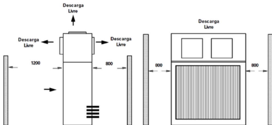
Fig. XVII 40 - Espaços sugeridos para manutenção e circulação de ar. Unidade condensadora TRCE 050 a 150.
