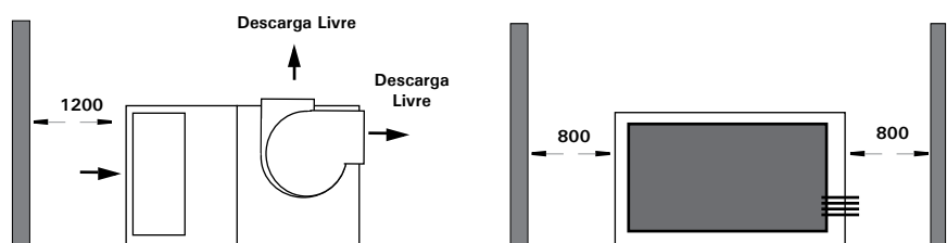
Fig. XVII-26 - Espaços sugeridos para manutenção e circulação de ar para os módulos serpentina e ventilador. (Gabinete Horizontal)
