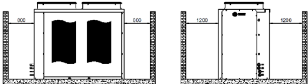
Fig. XVII 40 - Espaços sugeridos para manutenção e circulação de ar. Unidade condensadora TRCE 050 a 150.
