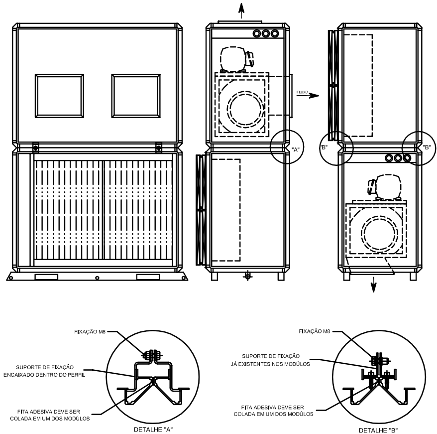
Fig. XVII-15 - Montagem Vertical 05 a 50 - DX/DL
