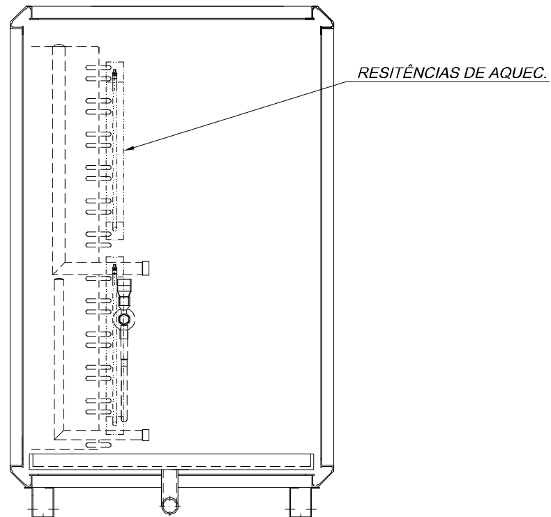
Fig. XVII-12 - Detalhes de Montagem do Módulo Serpentina 05 a 50
