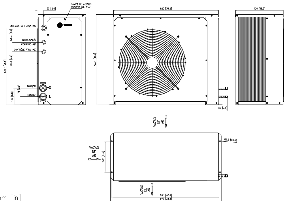
Fig. XVII-28 - Dimensional Unidades Condensadoras TRAE075 1 circuito
