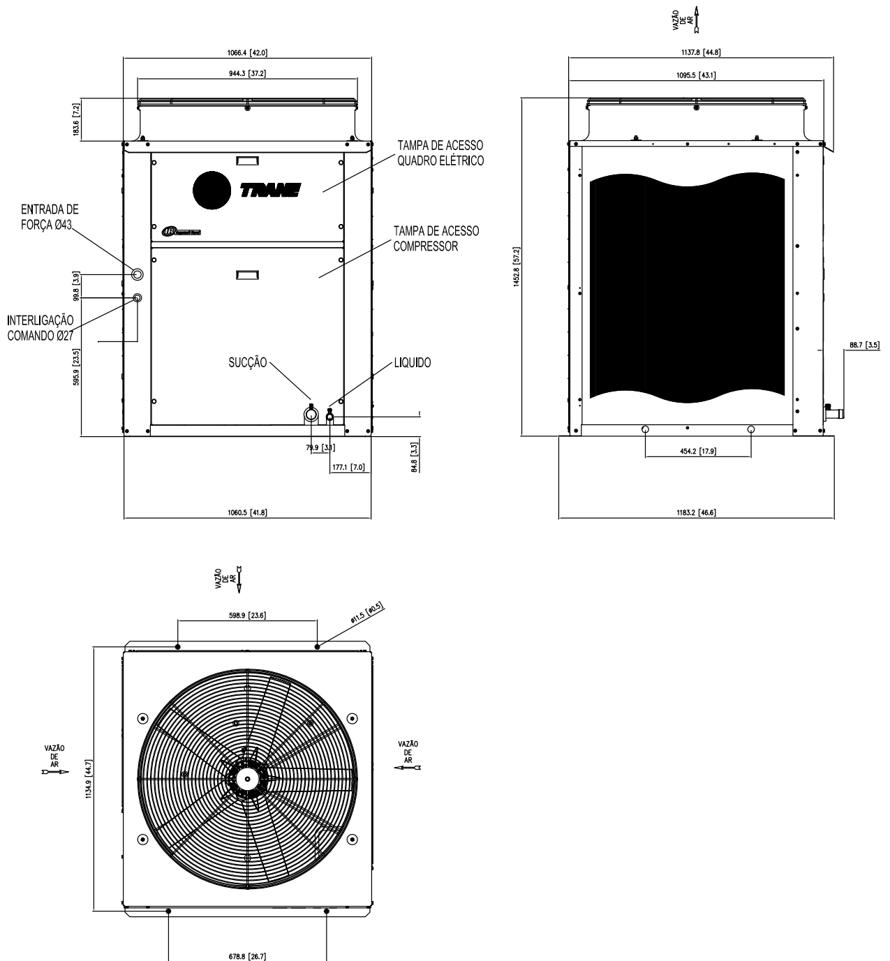
Fig. XVII-35 - Dimensional Unidades Condensadoras TRAE 250 - 1 circuito
