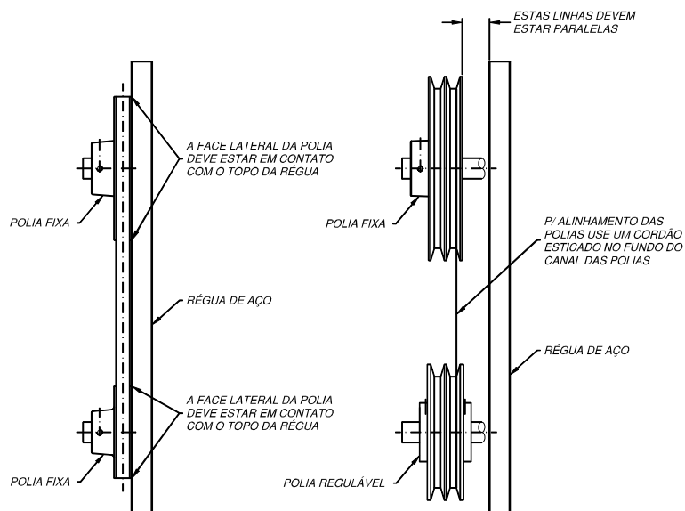
Fig. XV-03 - Alinhamento das correias
