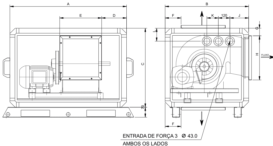
Fig. XVII-06 - Dimensões Módulo Ventilador 05 a 10 - Siroco e Limit Load
