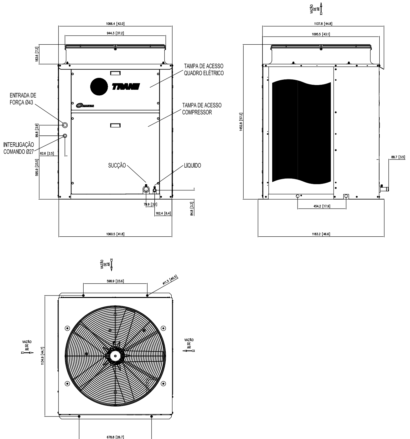
Fig. XVII-33 - Dimensional Unidades Condensadoras TRAE 200 - 1 circuito
