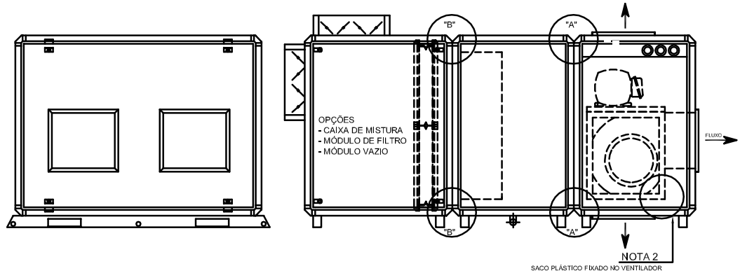
Fig. XVII-15 - Montagem Vertical 05 a 50 - DX/DL
