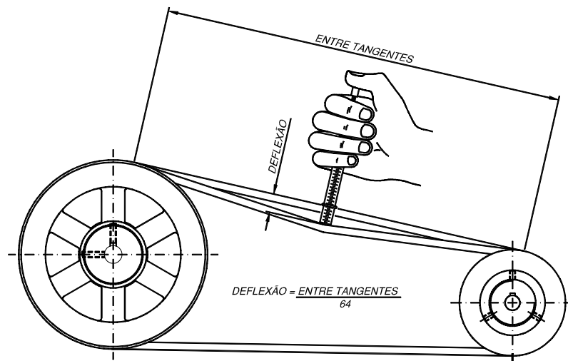
Fig. XV-02 - Ajuste da tensão da correia
