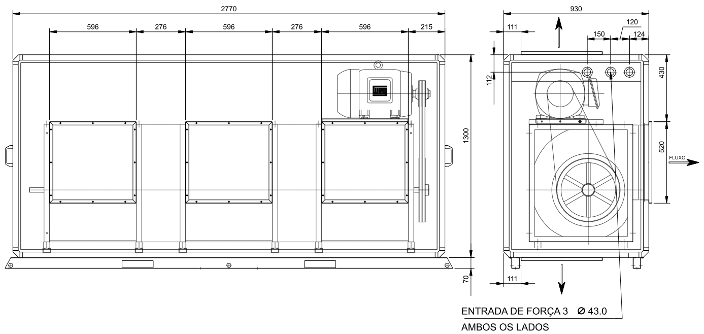
Fig. XVII-08 - Dimensões Módulo Ventilador 35/40/50 - Limit Load
