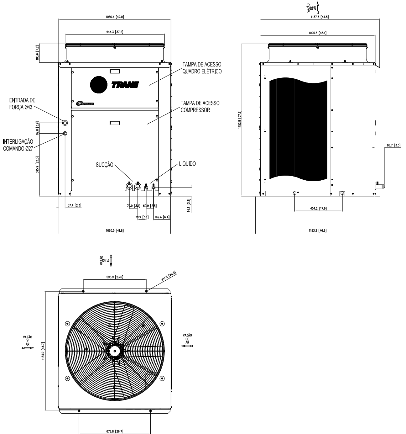
Fig. XVII-34 - Dimensional Unidades Condensadoras TRAE 200 - 2 circuitos
