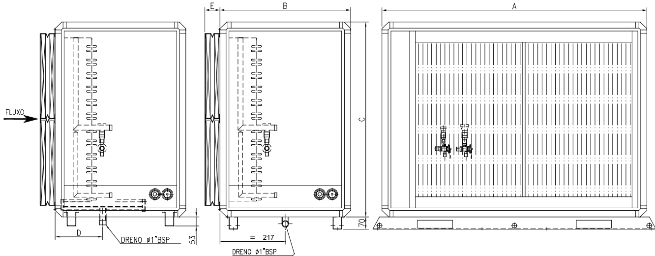
Fig. XVII-09 - Dimensões Módulo Serpentina 05 a 35
