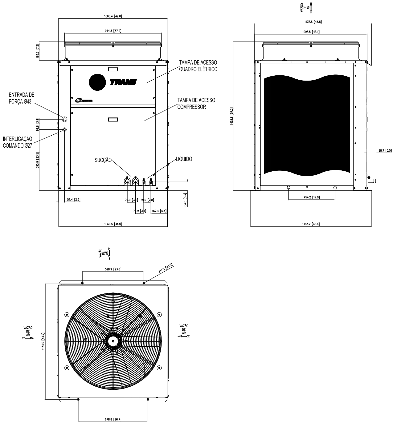
Fig. XVII-36 - Dimensional Unidades Condensadoras TRAE 250 - 2 circuitos
