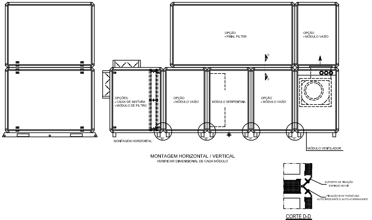
Fig. XVII - 18 - Montagem Horizontal com Final Filter
