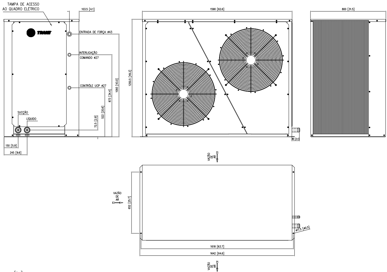
Fig. XVII-31 - Dimensional Unidades Condensadoras TRAE 150 - 1 Circuito
