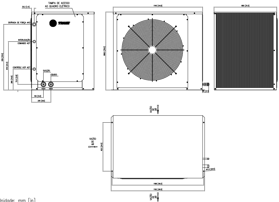
Fig. XVII-30 - Dimensional Unidades Condensadoras TRAE 100 - 2 circuitos
