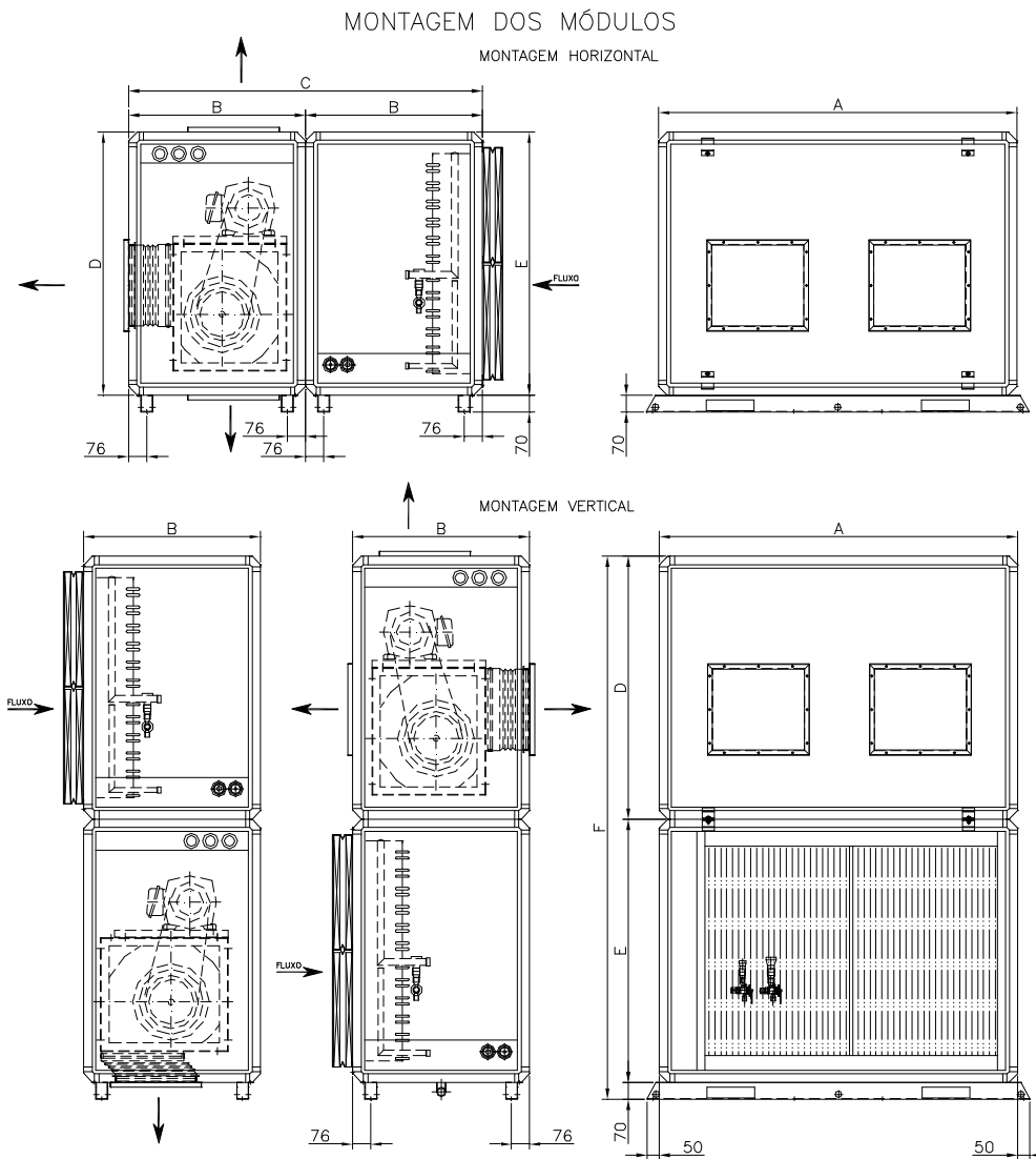
Fig. XVII-13 - Montagem dos Módulos Ventilador e Serpentina 05 a 50
