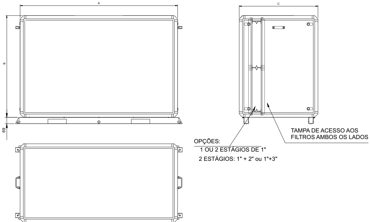
Fig. XVII-21 - Cotas Caixa de Mistura Sem Dampers dos Módulos 05 a 50 (1 ou 2 estágios de 1", 2 estágios 1" + 2", 2 estágios de 1" + 3")
