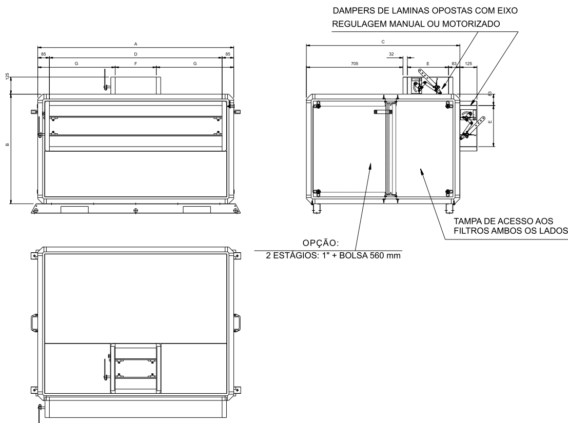
Fig. XVII-20 - Cotas Caixa de Mistura dos Módulos 05 a 50 (2 Estágios: 1" + Bolsa 560mm)
