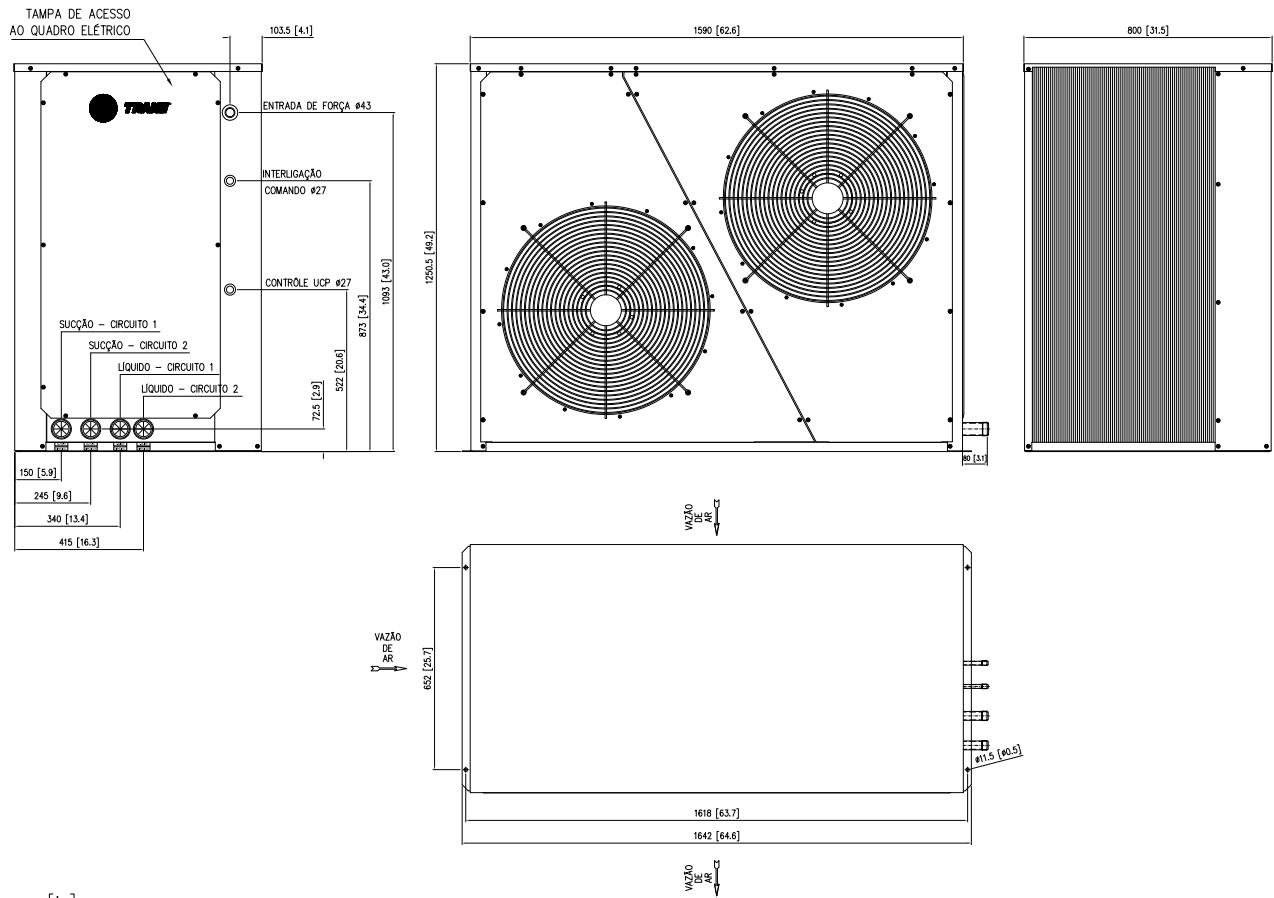
Fig. XVII-32 - Dimensional Unidades Condensadoras TRAE 150 - 2 Circuitos
