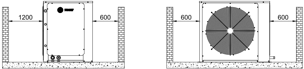
Fig. XVII 39 - Espaços para Manutenção e Circulação de Ar - TRAE
