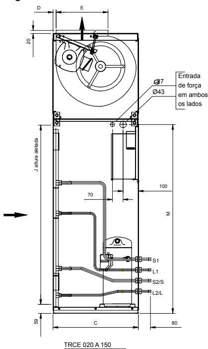
Fig. XVII 37 - Dimensional Conexões TRCE
