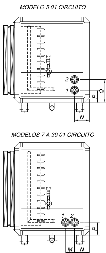
Fig. XVII-10 - Circuitos de Refrigeração do Módulo Serpentina 05 a 30
