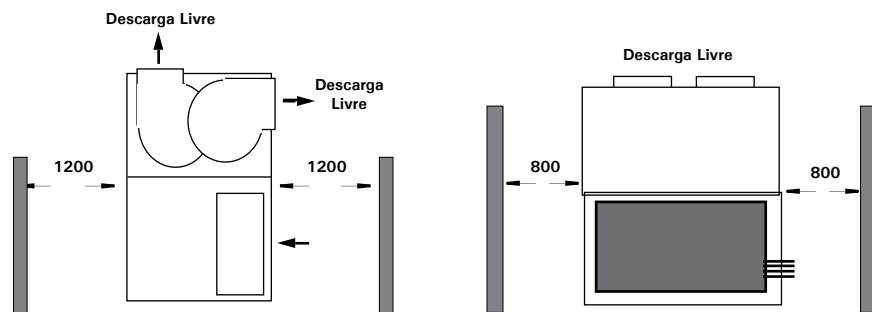
Fig. XVII-25 - Espaços sugeridos para manutenção e circulação de ar para os módulos serpentina e ventilador. (Gabinete Vertical)
