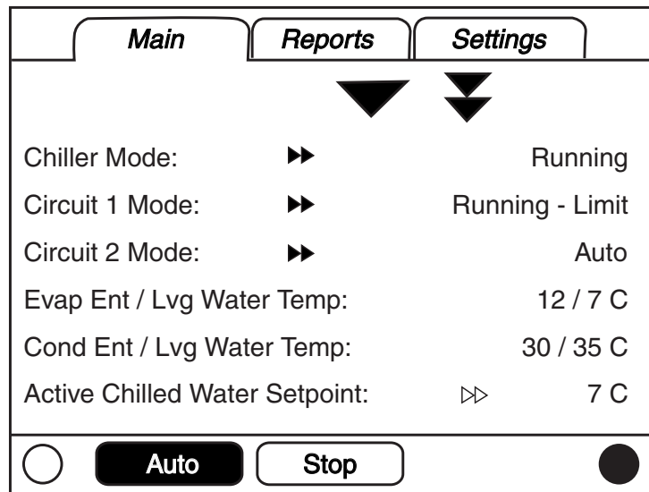
Рисунок 7 - Основное окно
